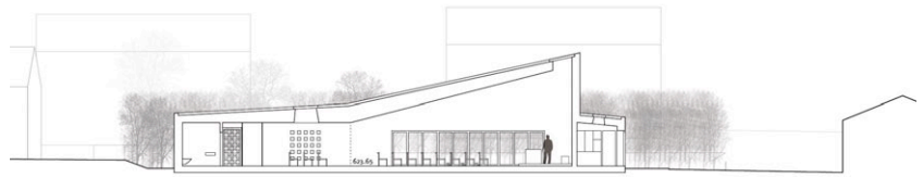
Längsschnitt
